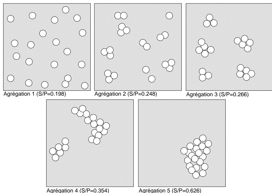
Fig. 2.8: Représentation schématique des indices d'agrégation; les cercles représentent les individus de l'espèce considérée. Le rapport Surface/Périmètre est calculé à partir des fragments de la population (groupes d'individus contigus).
