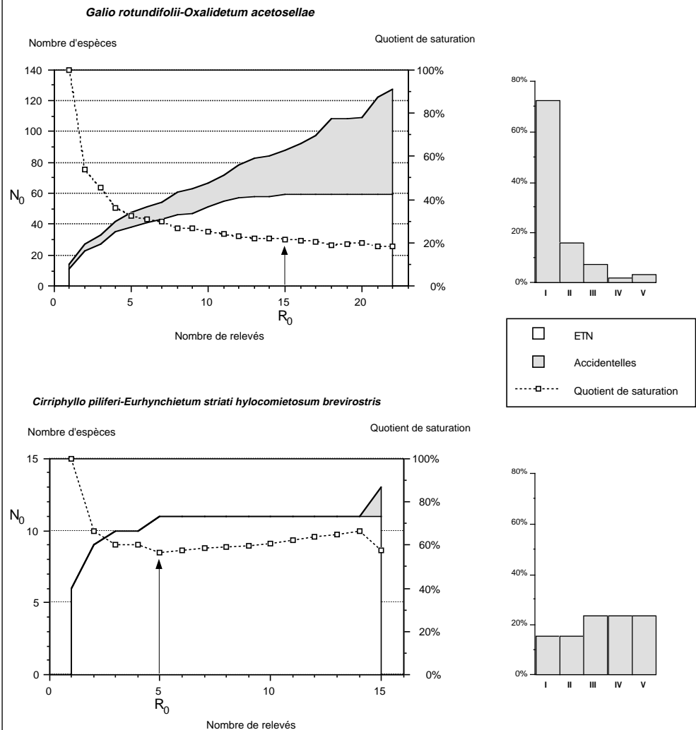
Fig. 3.2: Diagrammes d'homotonité et histogrammes de fréquences de deux syntaxons élémentaires.
